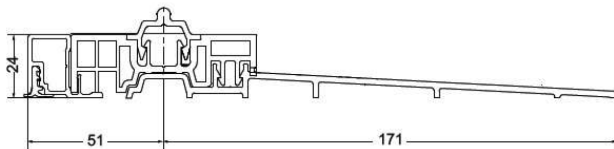
Sezione soglia ad incasso da 67 mm
