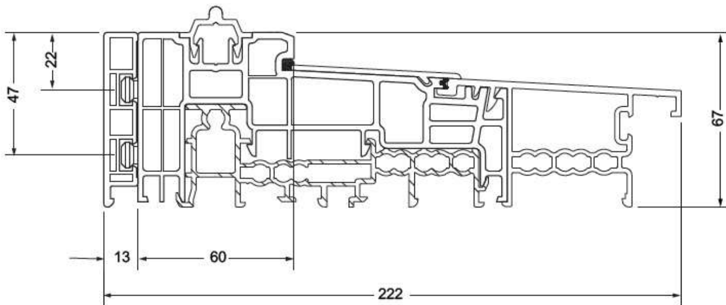
Sezione soglia ad incasso da 67 mm
